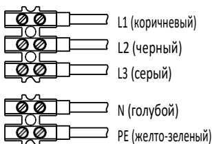
Трехфазное исполнение
