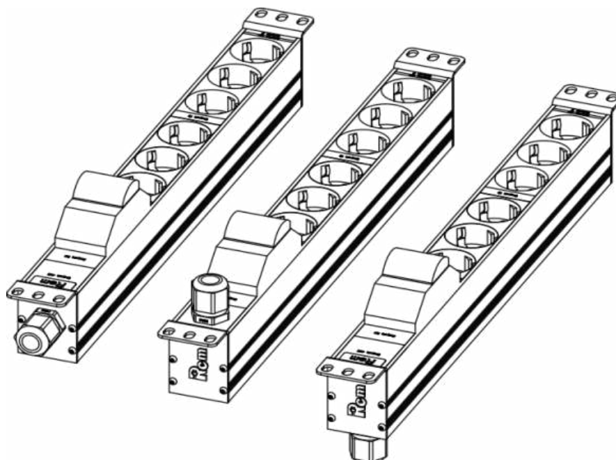
Рис. 1. Варианты монтажа кабельных вводов
