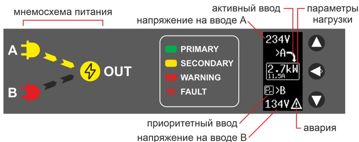
Рис. 9. Внешний вид модуля АВР
