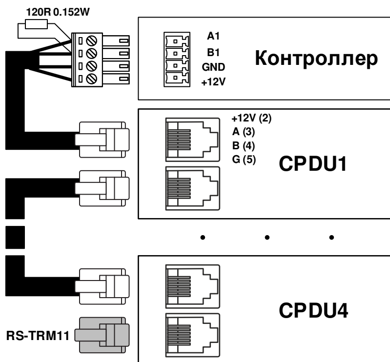
Рис.7. Схема подключения CPDU
