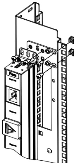
Рис. 3. Порядок монтажа вертикальных блоков
