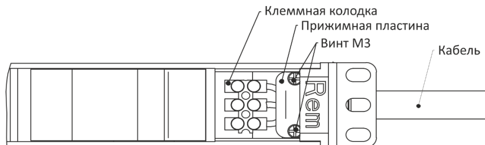
Рис. 5. Вид спереди на PDU в области клеммной колодки со снятой заглушкой
