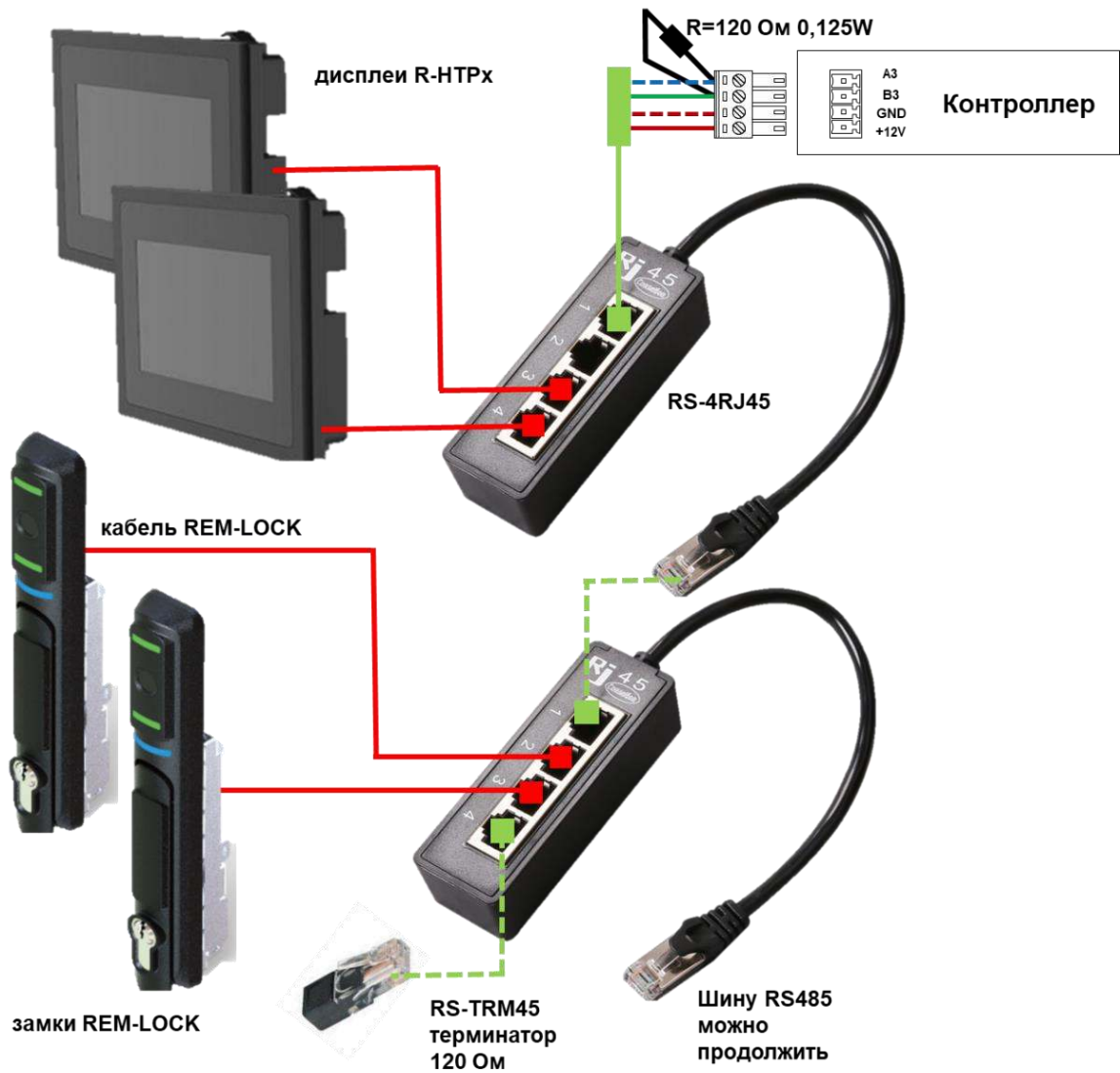
Рис. 6. Рекомендованная схема организация шины RS-485 при суммарной длине L<20м Рекомендованное подключение проводов RS-485 к разъёму RJ45
