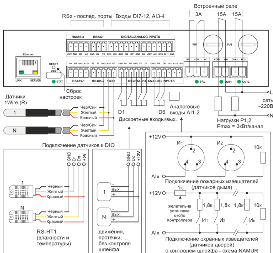
Рис. 6.1.1 Схема подключения датчиков и внешних устройств PDU 2
