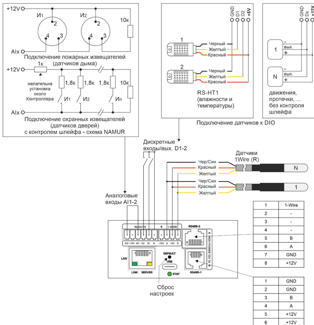
Рис. 6.1.3 Схема подключения датчиков и внешних устройств к PDU4
