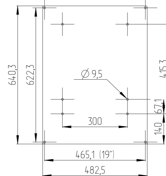
Панель ПМ-19"-15U (ПМ-19-15)
