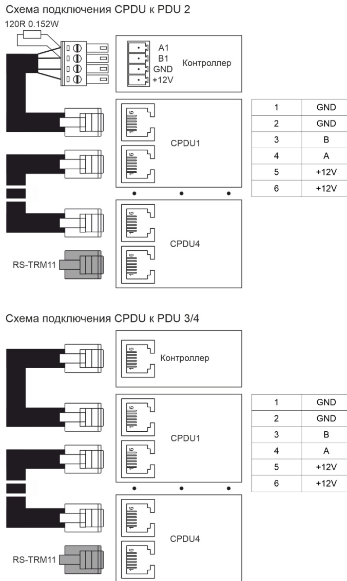
Рис. 6.9 - Схема подключения CPDU
