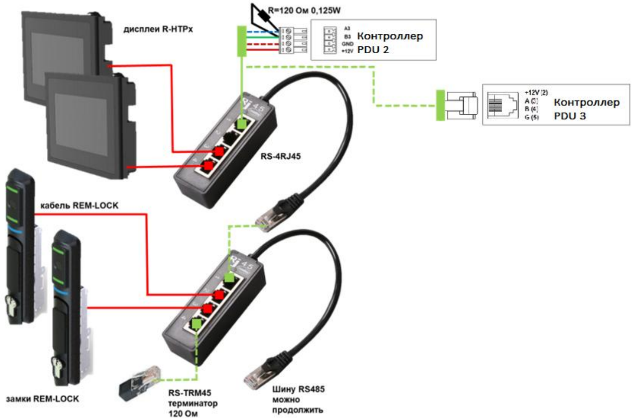
Рис. 6.8 - Рекомендованная схема организация шины RS-485 при суммарной длине L <20м
