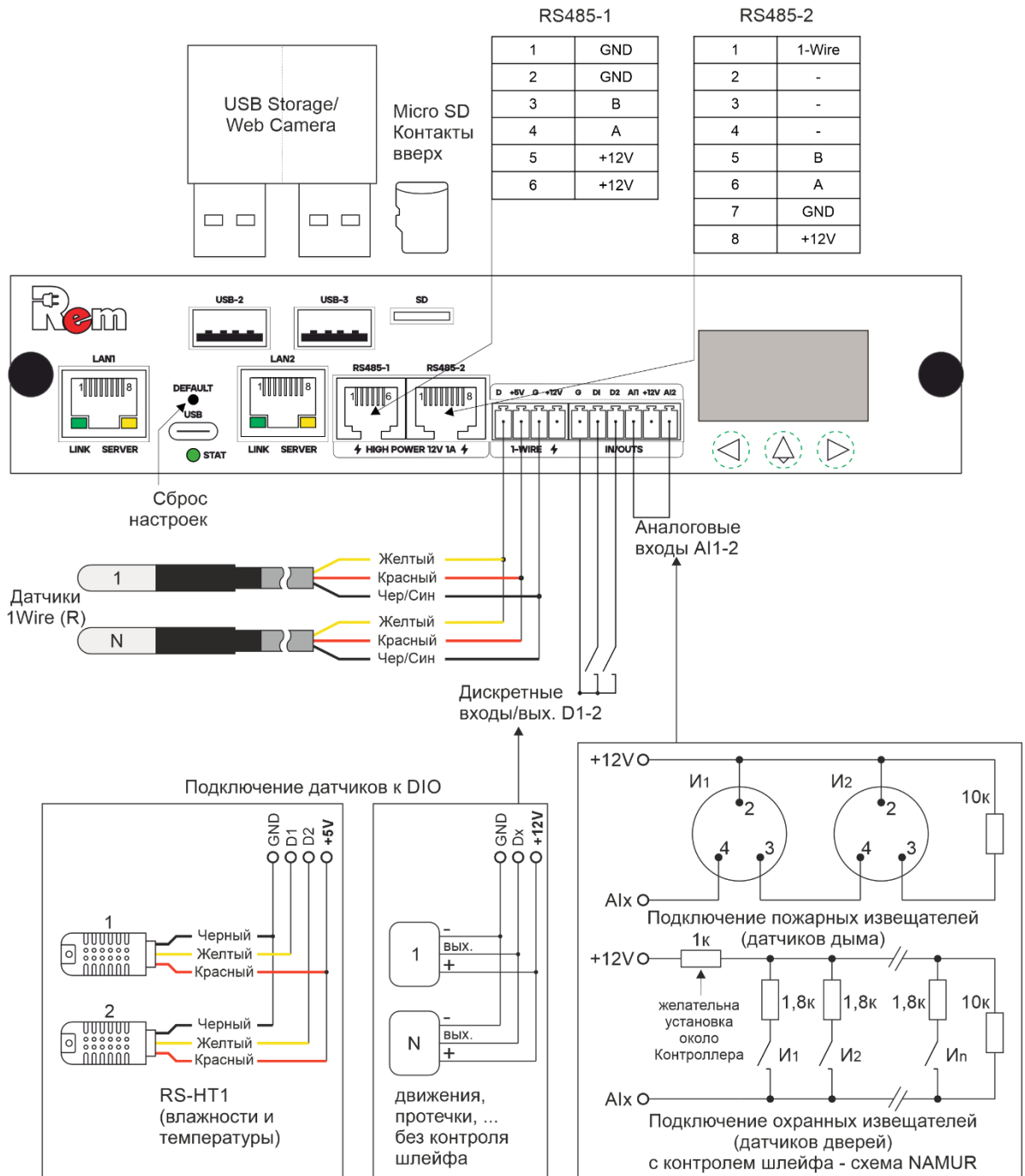
Рис. 6.1.2 Схема подключения датчиков и внешних устройств к PDU3
