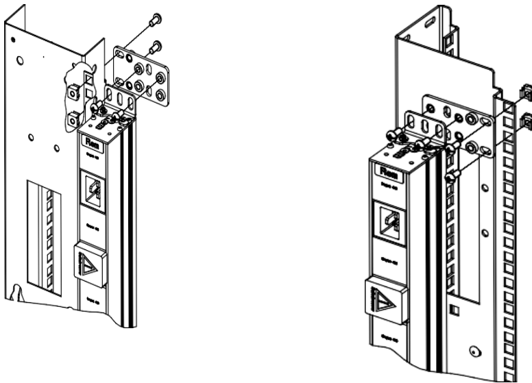
Рис. 5.3 - Порядок монтажа вертикальных блоков
