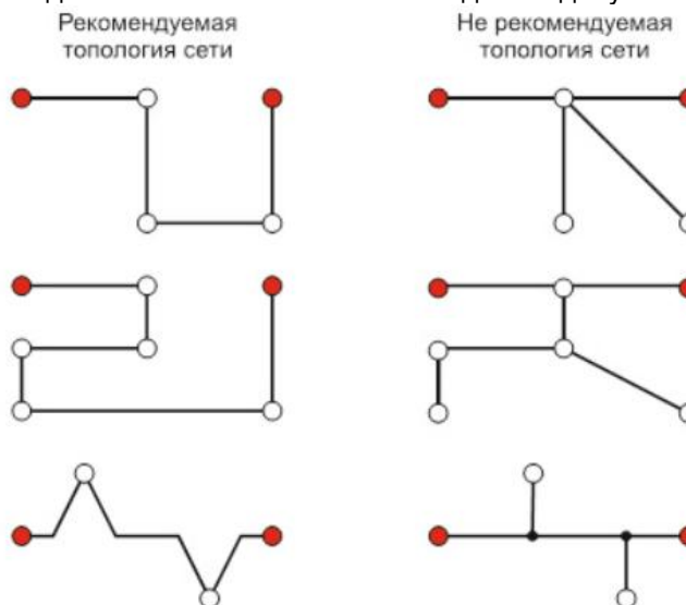
○ Узел сети RS-485, ● Узел с подключенным согласующим резистором ("терминатором").
