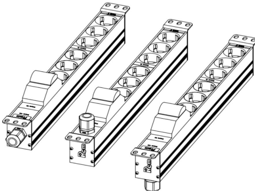
Рис. 5.1 - Варианты монтажа кабельных вводов
