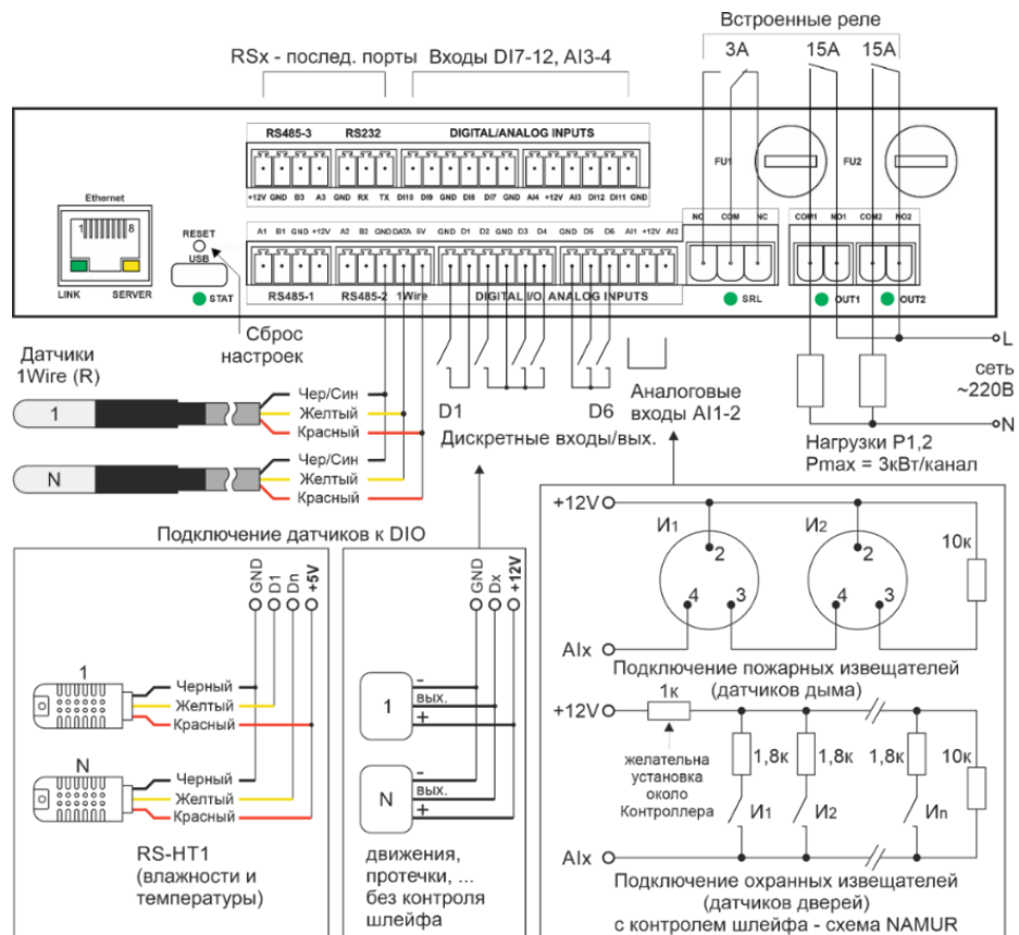
Рис. 6.1.1 Схема подключения датчиков и внешних устройств PDU 2
