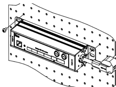
Рис. 5.2 - Порядок монтажа горизонтальных блоков
