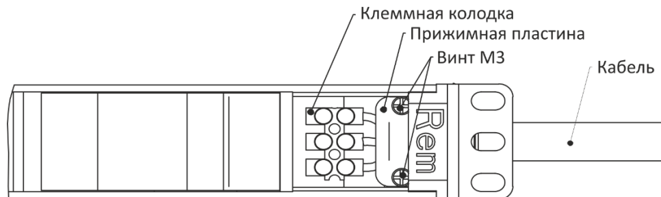
Рис. 6.4 - Вид спереди на PDU в области клеммной колодки со снятой заглушкой
