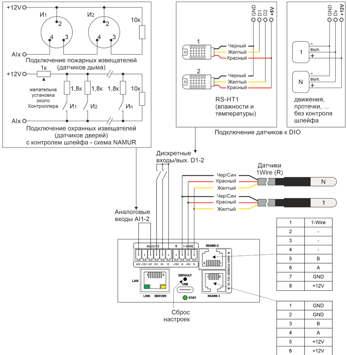
Рис. 6.1.3 Схема подключения датчиков и внешних устройств к PDU2S и PDU4
