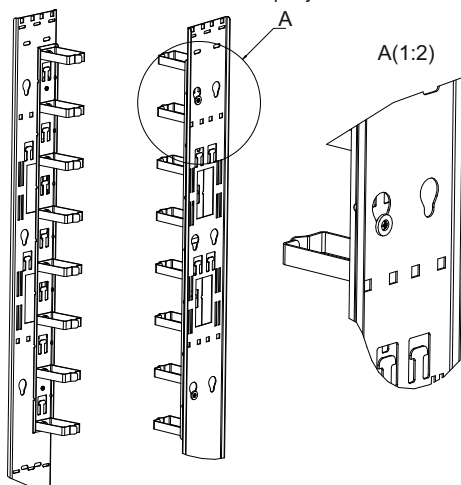
Рисунок 1. Установка изделия
