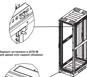
Вариант установки в ШТК-М для боковой обшивки
