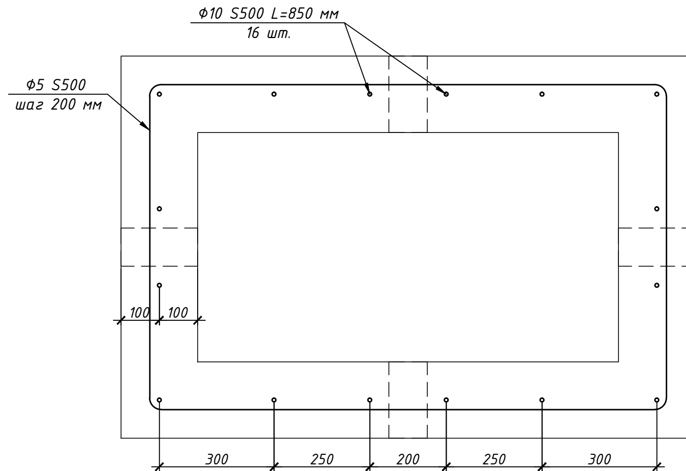
3-3 (армирование)
