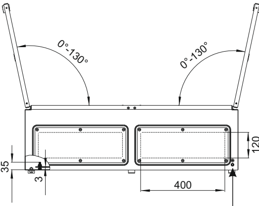
Элемент для подключения заземления, болт М8
