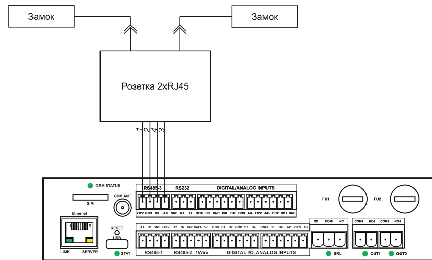
Рисунок 3. Схема подключения цифрового замка к контроллеру REM
