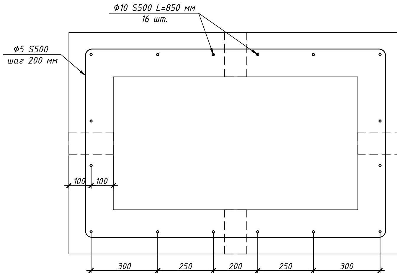
3-3 (армирование)
