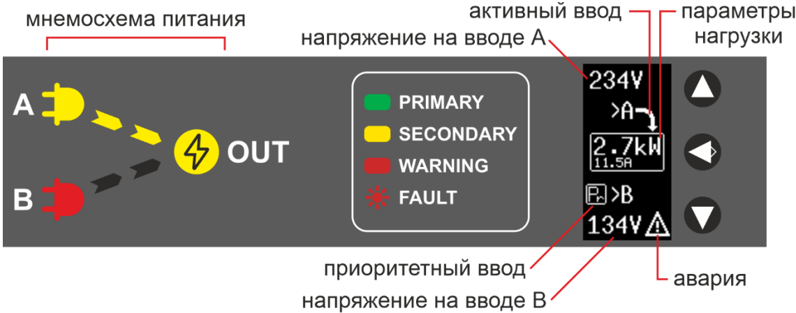
Рис. 7.7 - Внешний вид модуля АВР
