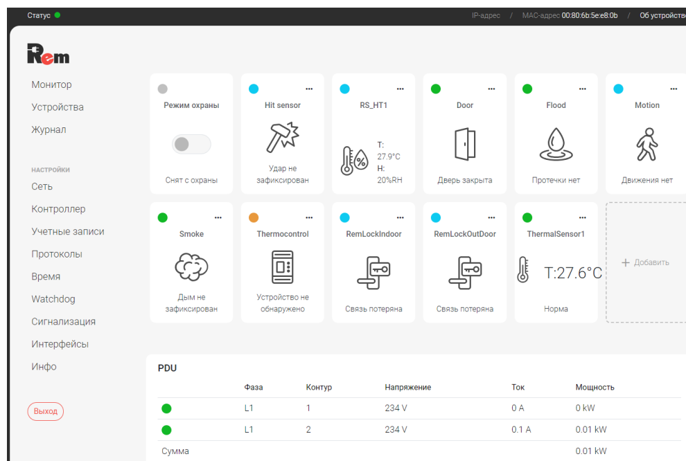
Рис. 8.1.2.2 - Окно «Монитор» WEB-Интерфейса
