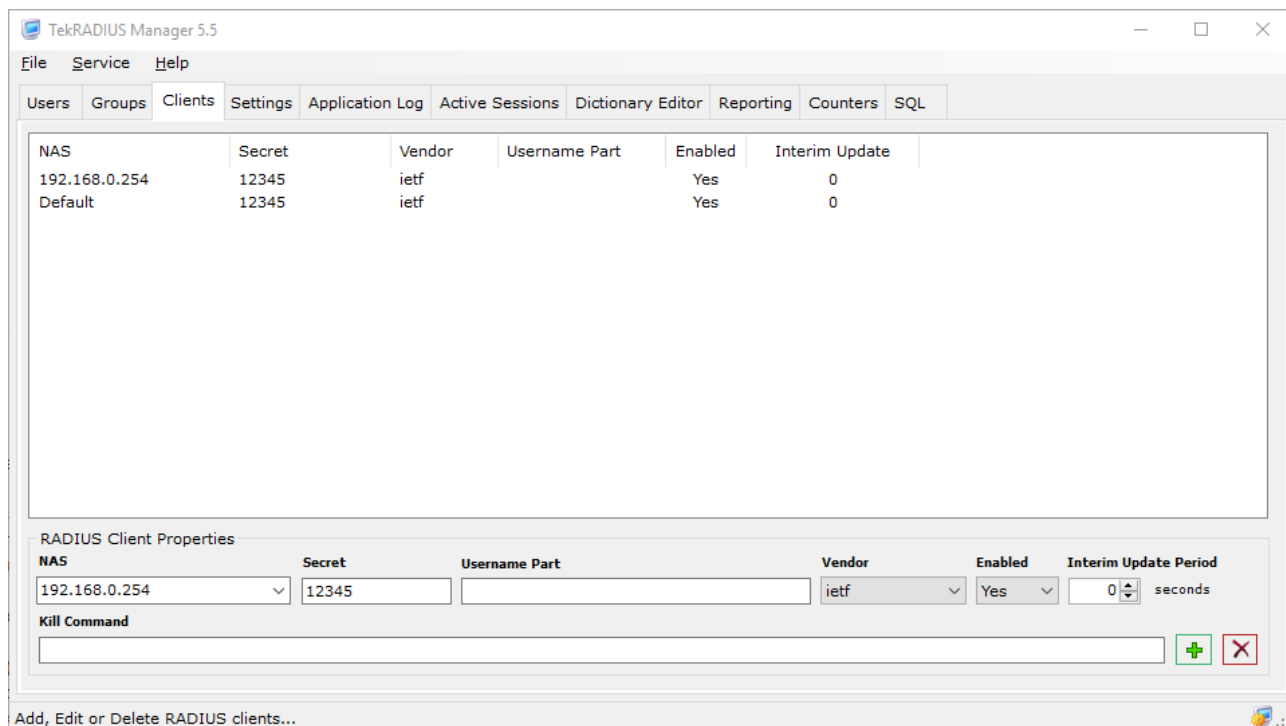
Рис. 8.14.1.1 - Окно добавления клиента tekRADIUS
