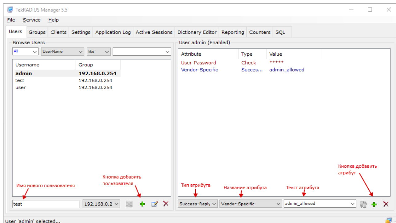
Рис. 8.14.1.2 - Окно добавления пользователя tekRADIUS
